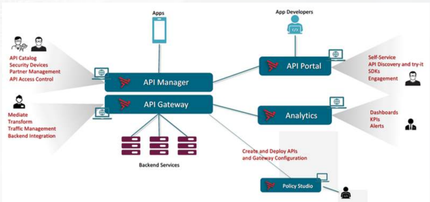
Mô hình tổng quan khối các ứng dụng của Axway API Management
